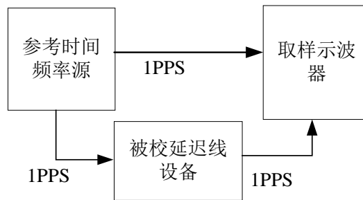
图 4 时延分辨力测量仪器连接示意图
