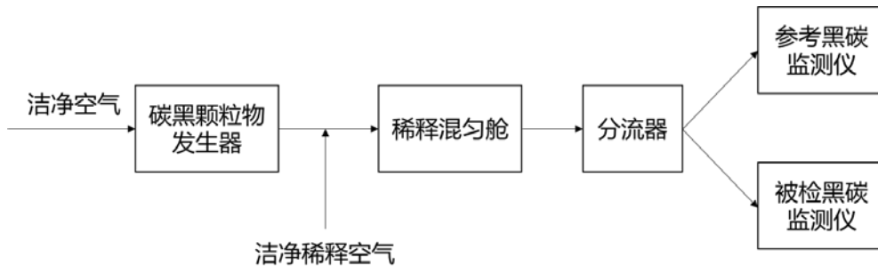
图 A.1 碳黑颗粒物标准装置结构示意图
