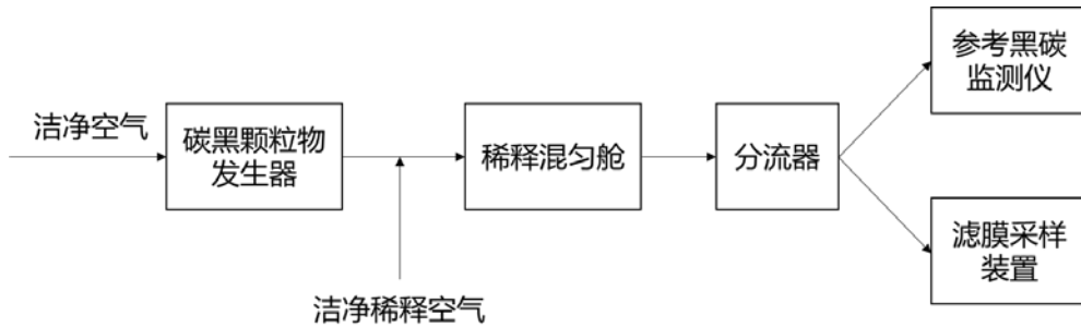
图 B.1 参考黑碳监测仪校准示意图
