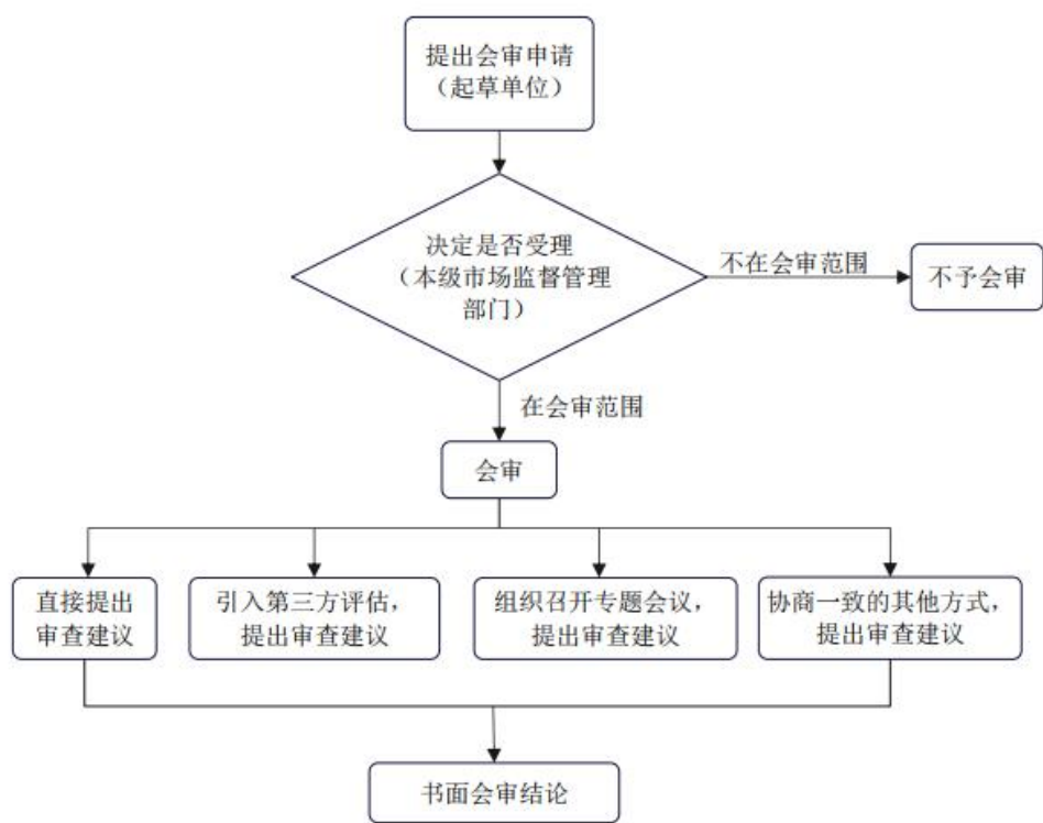
图 C.1 会审程序流程图
