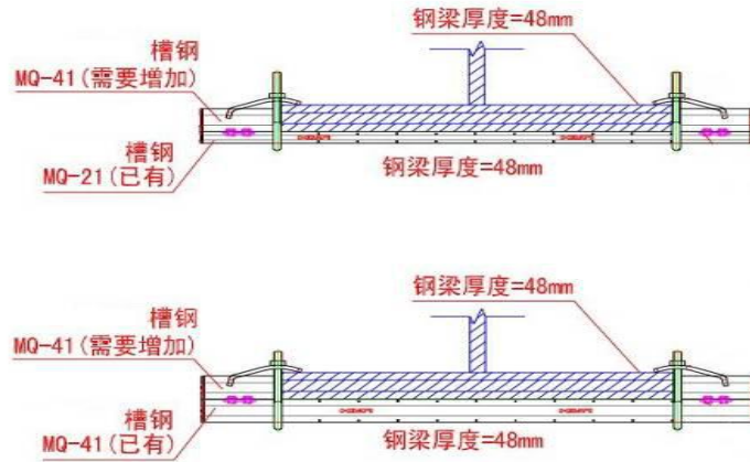
图 3.4.3-7 钢梁翼缘 48mm 梁夹固定示意图
