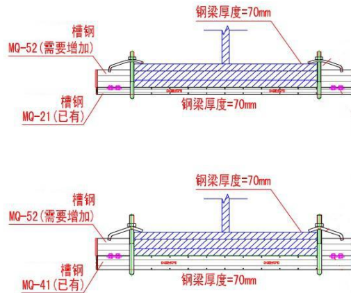
图 3.4.3-8 钢梁翼缘 70mm 梁夹固定示意图
