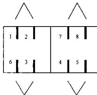
4.4.6-3 7类和7a类插座连接（正视）方式2
