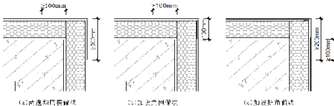
图 4.4.11-1 阳角处玻纤网做法示意图
