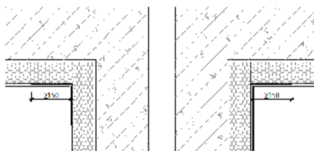
图 5.4.13-2 阴角处玻纤网做法示意图
