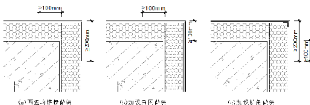
图 5.4.13-1 阳角处玻纤网做法示意图
