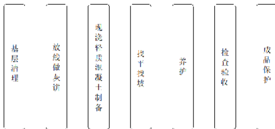
图 10.4.1-2 屋面保温现浇施工工艺流程
