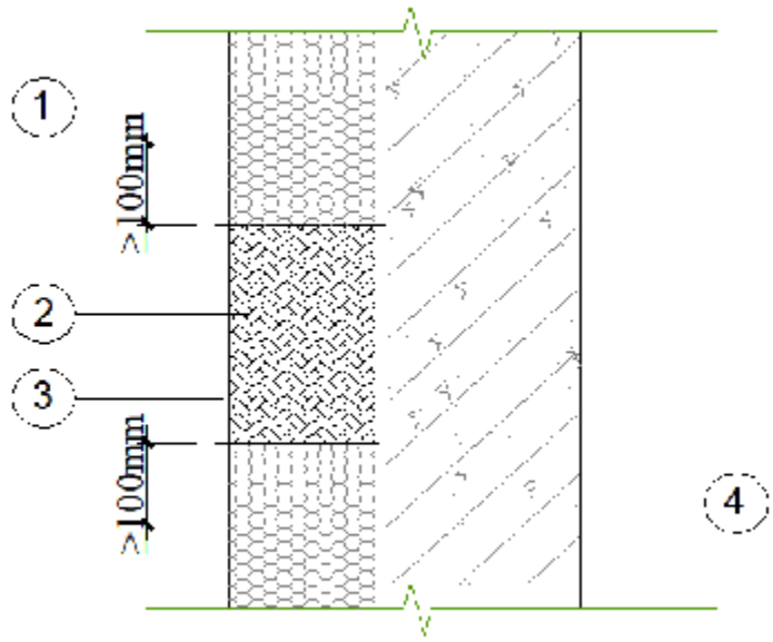
图 5.4.11-2 玻纤网格布搭接示意图
