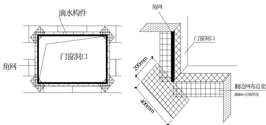
图 5.4.11-1 门窗洞口增强处理示意图
