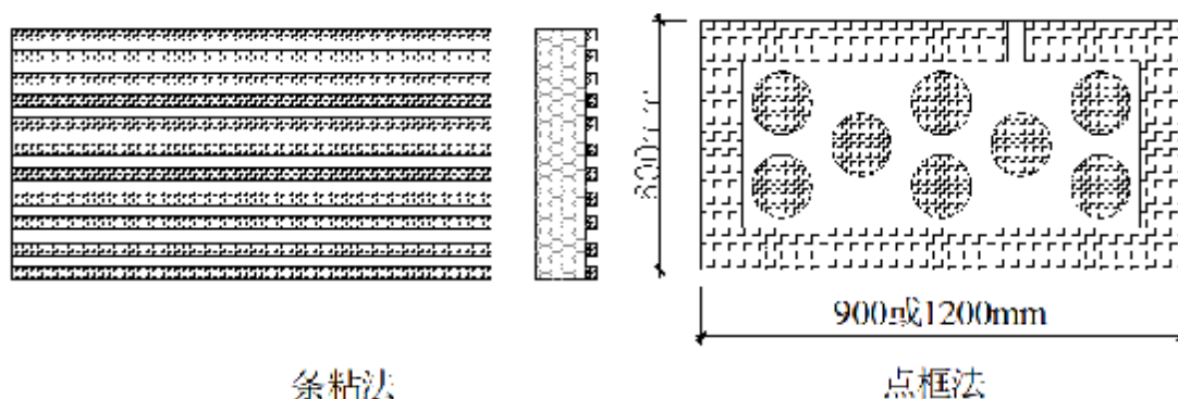
图 5.4.9-2 条粘法、点框法示意图
