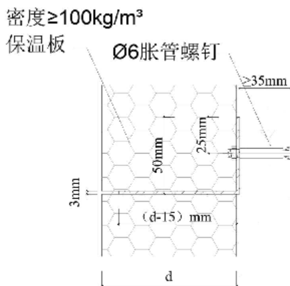
图 3.4.5 托架安装示意图
