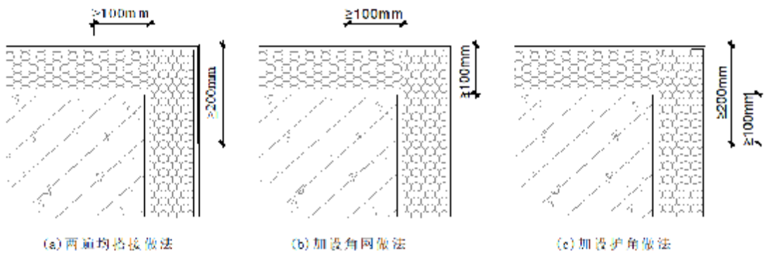
图 3.4.6-1 阳角处玻纤网做法示意图
