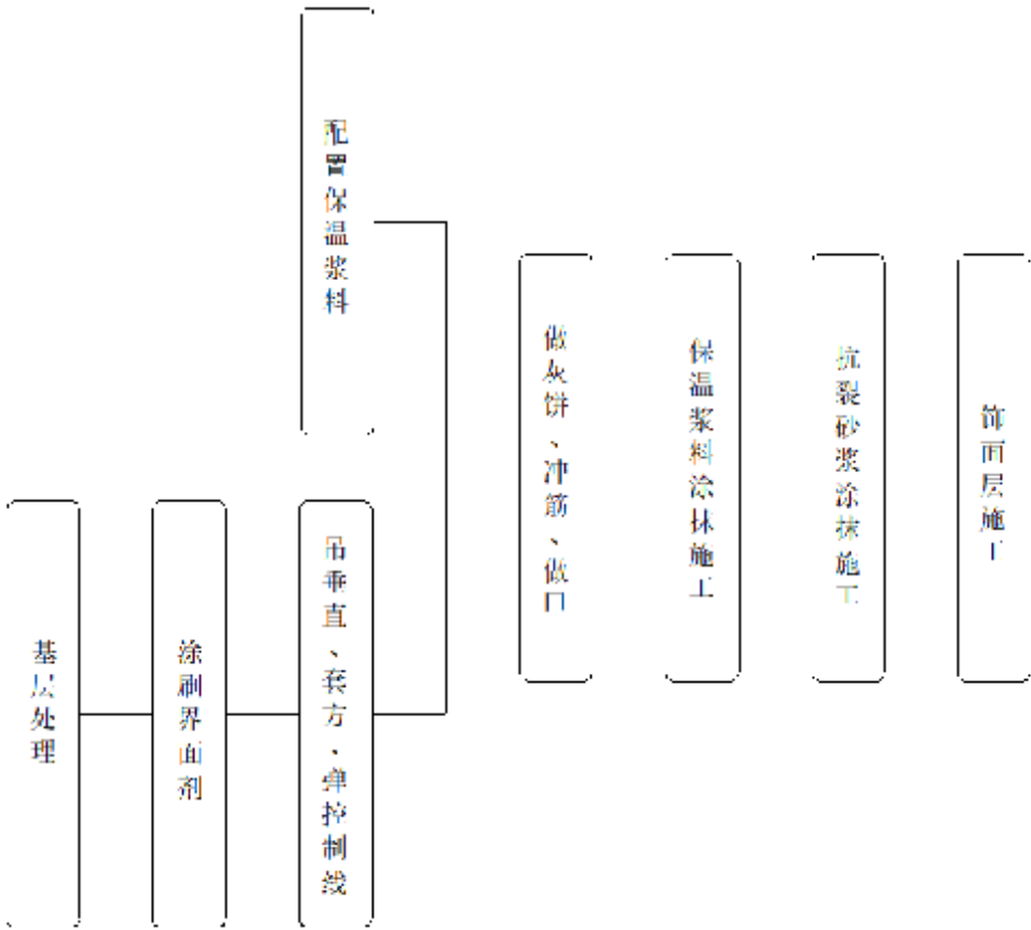
图 8.4.1 内墙保温浆料施工工艺流程
