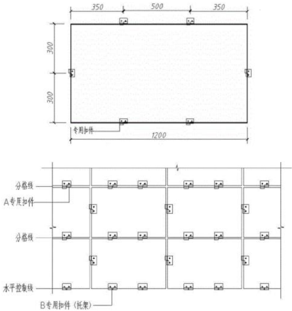
图 6.4.8-2 锚固件安装示意图
