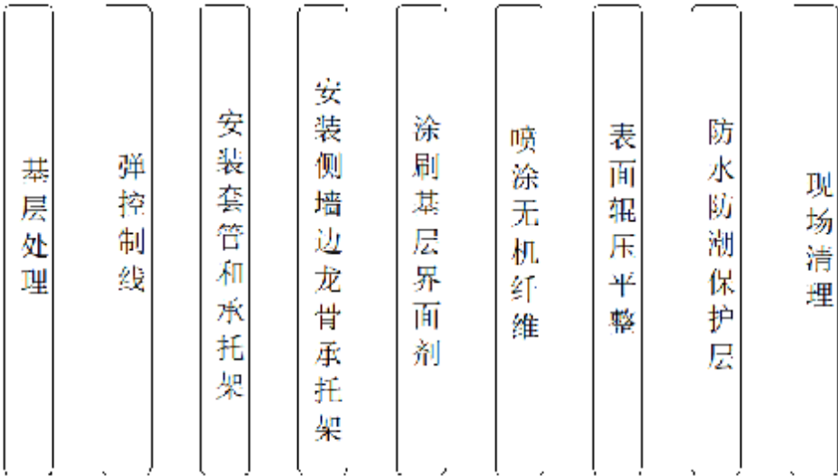
图 12.4.1-2 无机纤维喷涂厚度 60mm 以上的施工工艺流程
