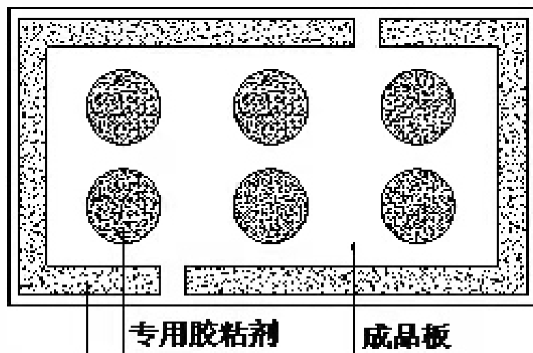
图 6.4.6 保温装饰板点框法粘贴示意图
