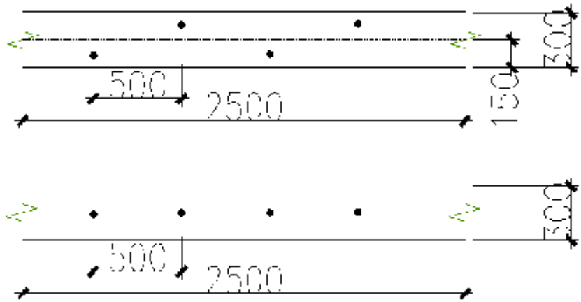
图 5.4.12-2 锚栓位置示意图
