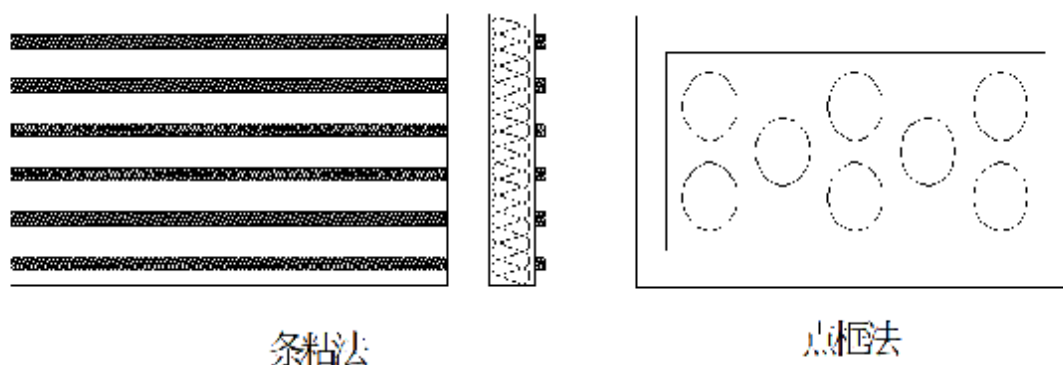
图 3.4.8-2 条粘法、点框法示意图
