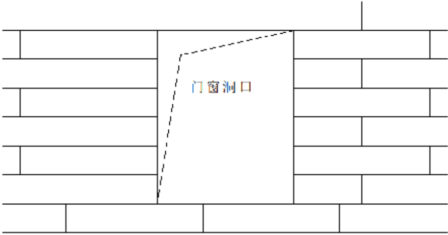
图 4.4.8-1 门窗洞口岩棉排布示意图
