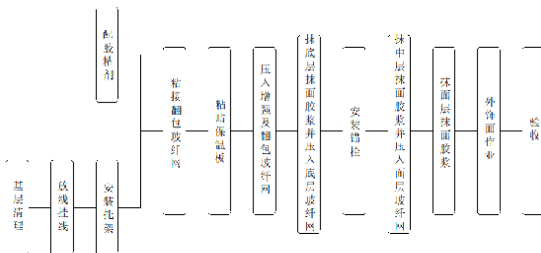
图 3.4.2 外墙 A 级保温材料双网构造保温施工工艺流程
