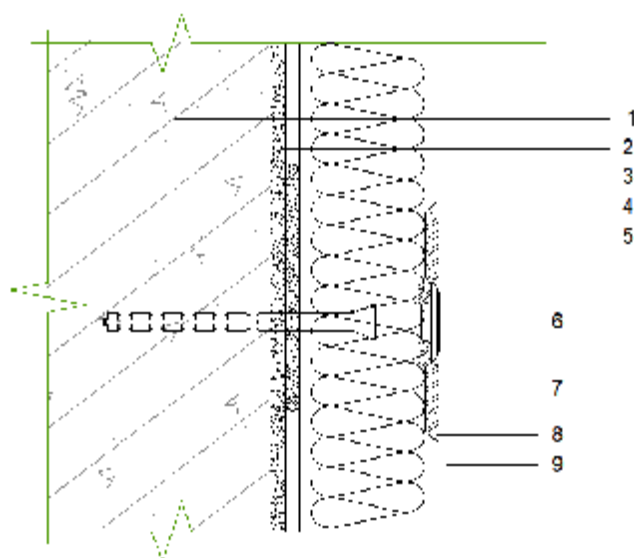
图 4.4.1 岩棉条锚盘压网单网构造示意
