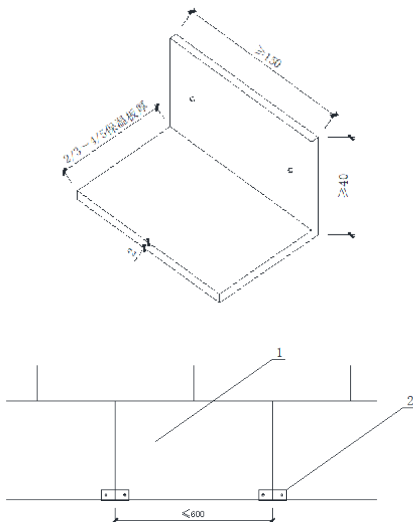
图 7.4.5 托架及安装示意 (单位: mm) 1—保温板; 2—托架
