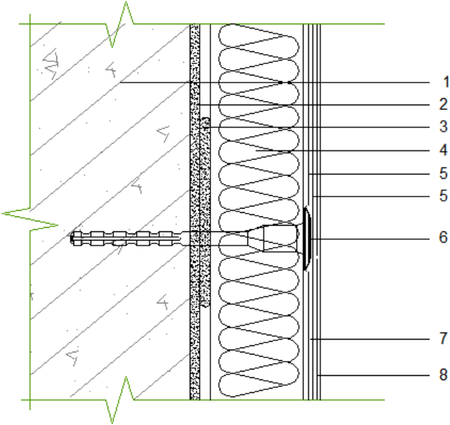
图 3.4.1 岩棉条或岩棉板锚盘压网双网构造
