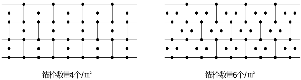
图 5.4.12-1 保温板（1200mm×600mm）排版及锚栓位置示意图
