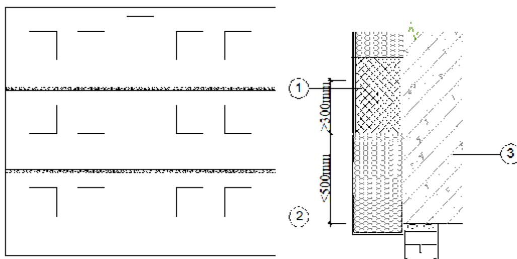
图 5.4.10-1 水平隔离带位置示意图
