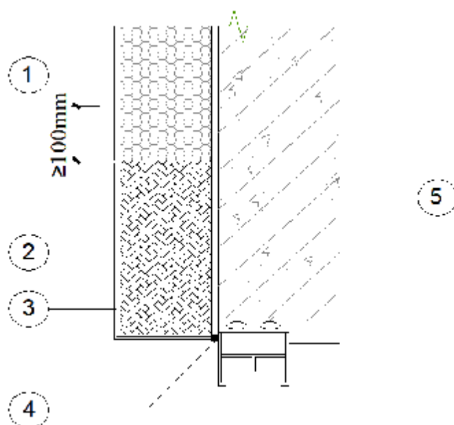
图 5.4.8 翻玻纤网格布做法
