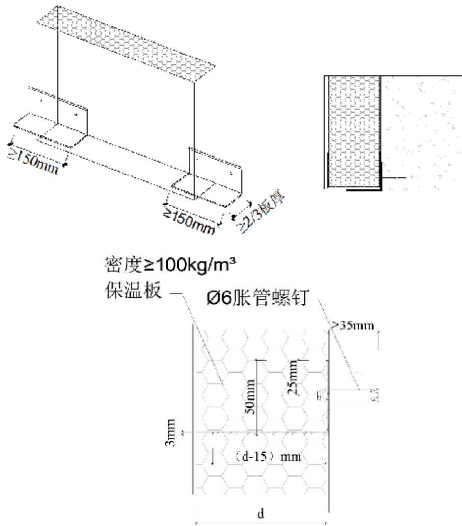
图 5.4.5 托架安装示意图
