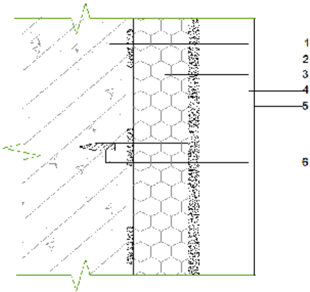
图 5.4.1 粘贴保温板薄抹灰外保温系统图 1-基层墙体；2-胶粘剂；3-保温板 4-抹面胶浆复合玻纤网；5-饰面层；6-锚栓
