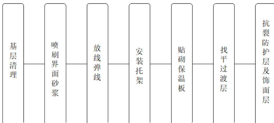
图 7.4.1 外墙保温板复合胶粉聚苯颗粒贴砌工艺流程
