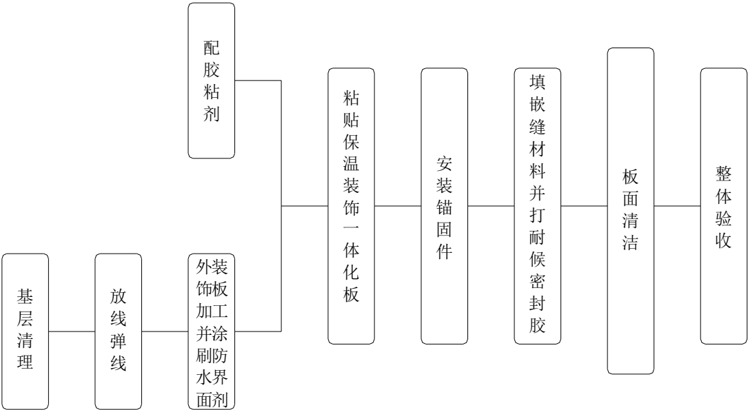
图 6.4.1 外墙保温装板施工工艺流程
