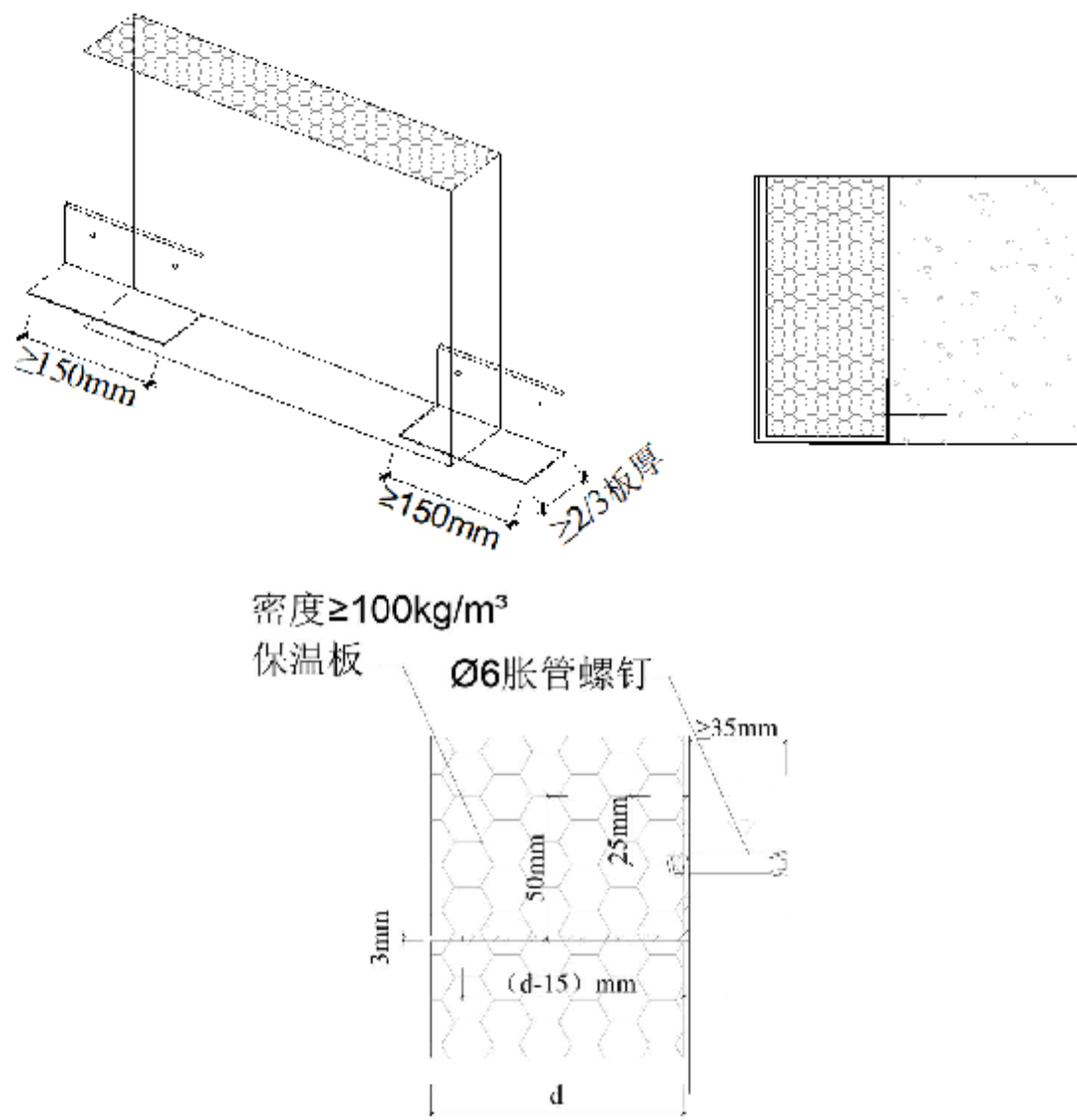
图 4.4.5 托架安装示意图
