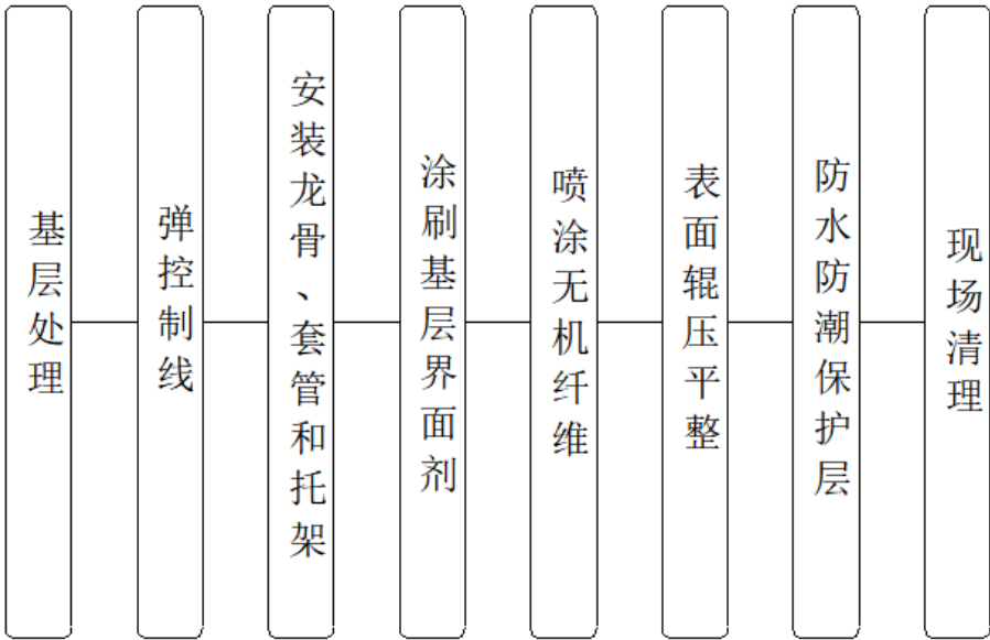
图 12.4.1-1 无机纤维喷涂厚度 60mm 以内的施工工艺流程
