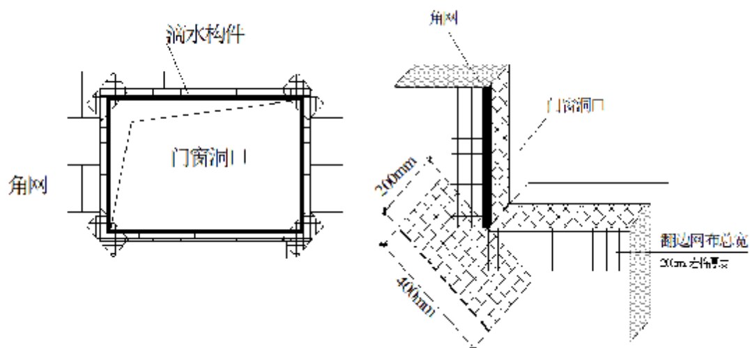
图 3.4.9 门窗洞口增强处理示意图
