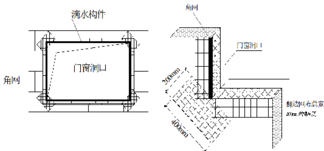
图 4.4.10 门窗洞口增强处理示意
