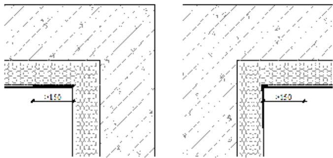
图 3.4.6-2 阴角处玻纤网做法示意图
