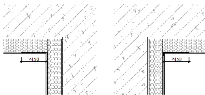
阴角处玻纤网做法示意图
