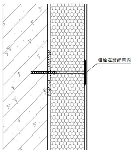
图 5.4.13-3 锚栓位置示意图
